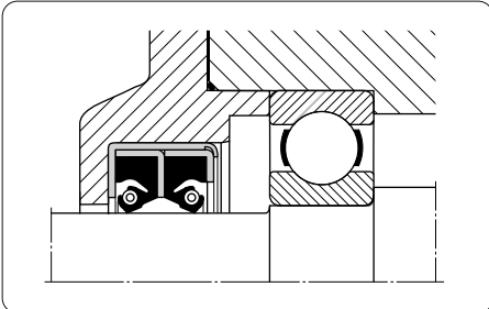
Fig 18. HDSD1 seal
