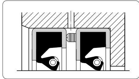
Fig 62. Spacer lugs
